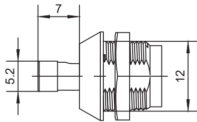
开启状态 Open state
