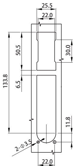
开孔尺寸 Panel cutout
