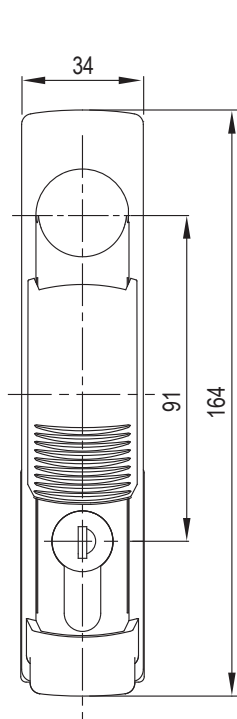
半圆柱 K333 相同钥匙 Alike K333 Profile Round Cylinder
