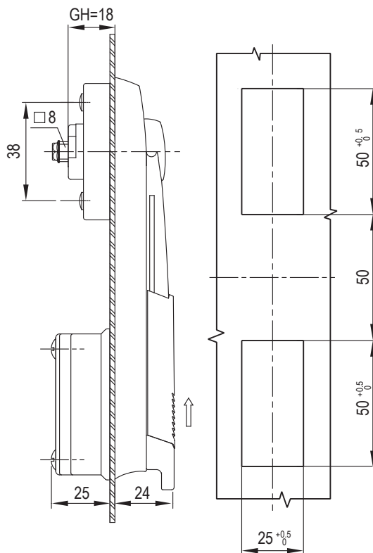
开孔尺寸 Panel Cutout
