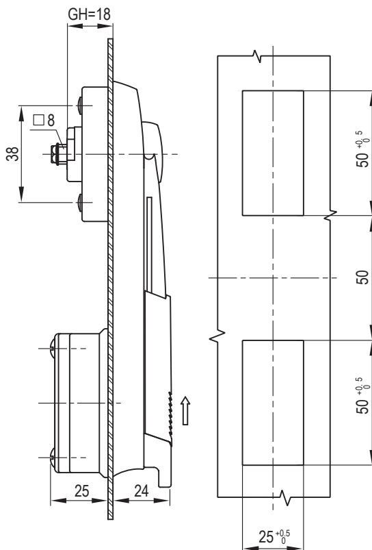
开孔尺寸 Panel Cutout
