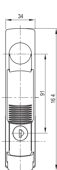
圆柱 K333 相同钥匙 Alike K333 Round Cylinder
