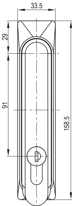
半圆柱 K333 相同钥匙 Alike K333 Prople Round Cylinder
