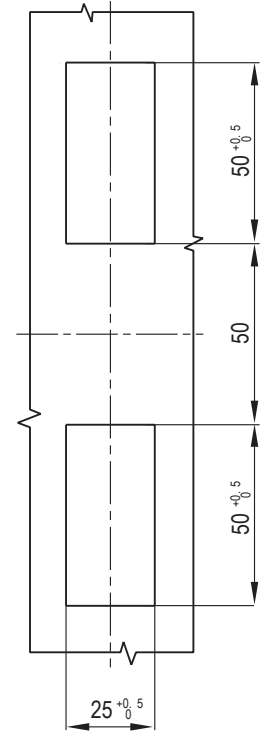
开孔尺寸 Panel Cutout
