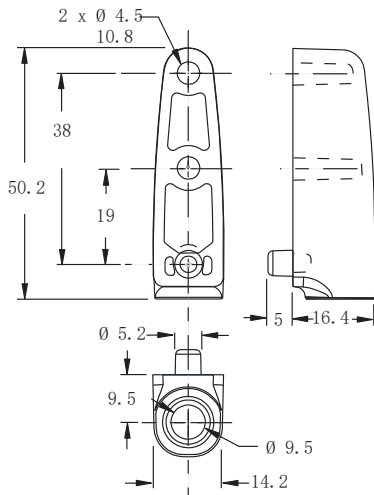
偏置固定 Offset Mount
