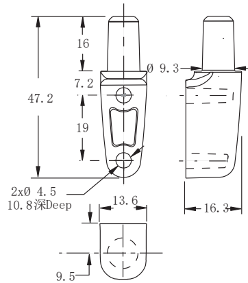
齐平固定 Flush Mount
