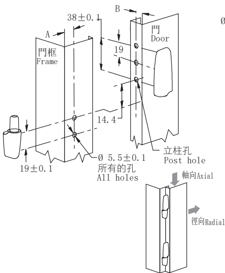
偏置固定 Offset Mount
