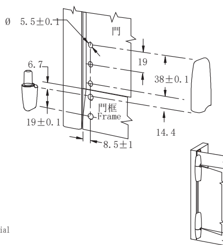
齐平固定 Flush Mount
