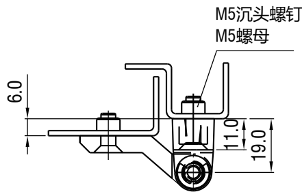
高度增加6MM型 Height:6mm higher
