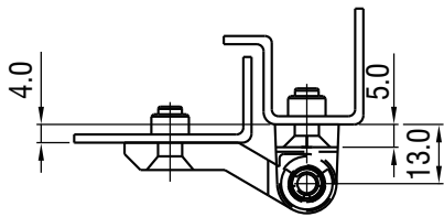
高度增加4MM型 Height:4mm higher
