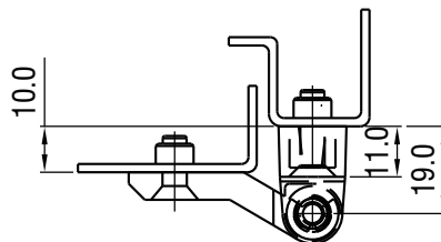
高度增加10MM型 Height:10mm higher
